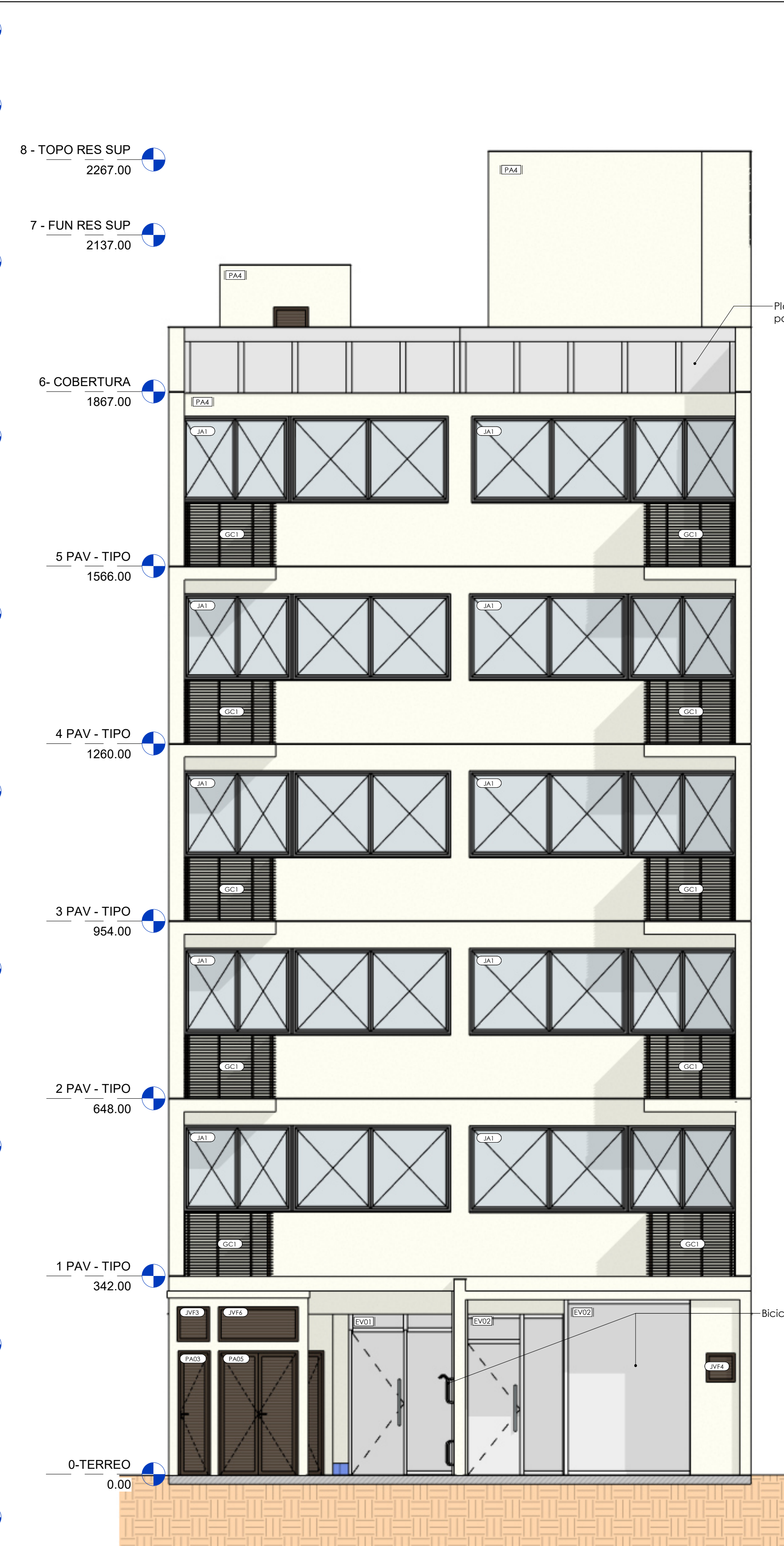
FACHADA FRENTE ESC: 1 : 50
