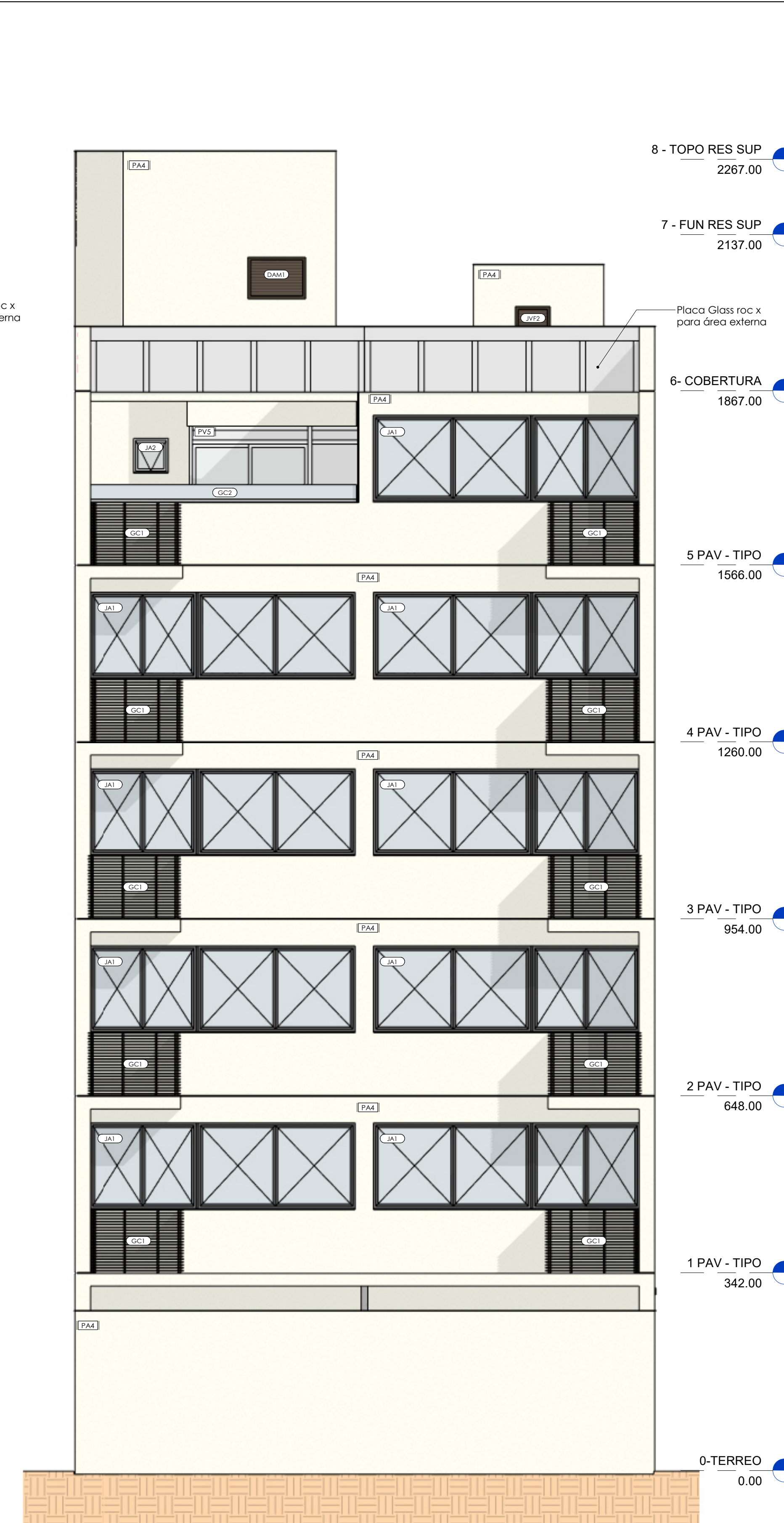
FACHADA POSTERIOR ESC: 1 : 50
