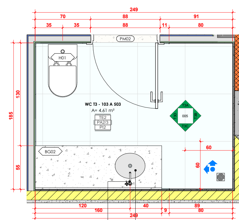
WC T03 ESC: 1 : 25
