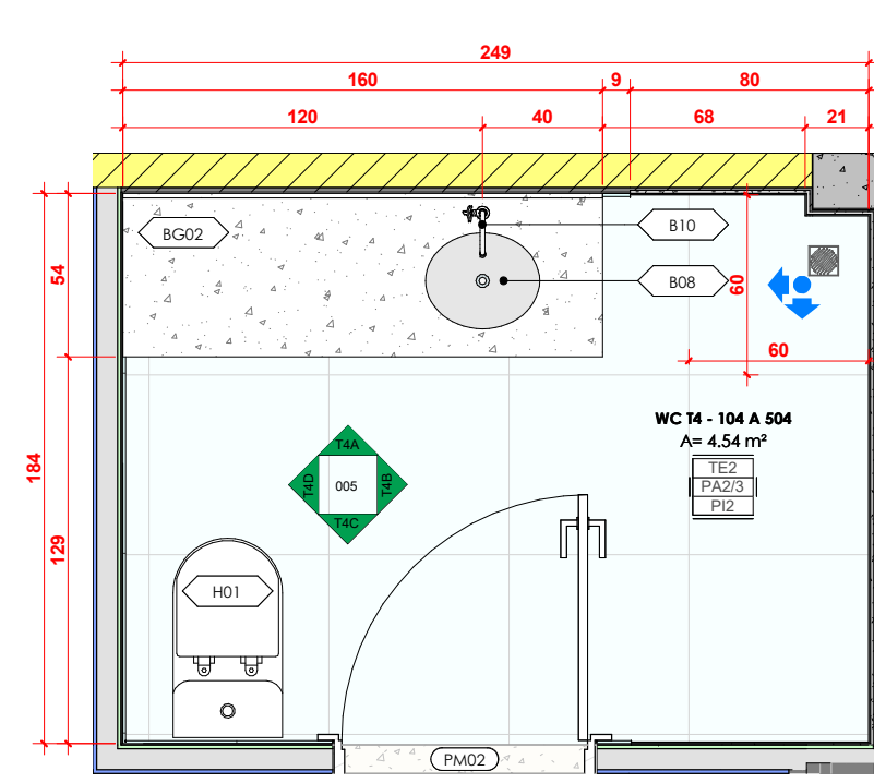
WC T04 ESC: 1 : 25
